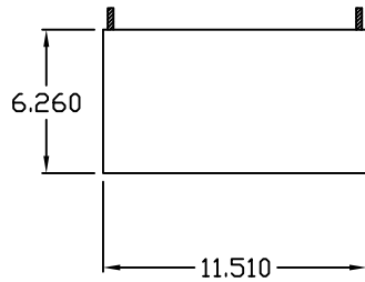
IQ1200VS IQ1500VS IQ1800VS FRONT VIEW
