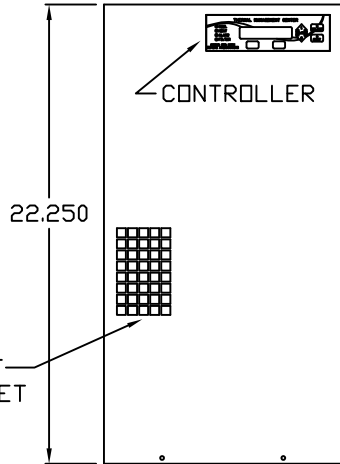
IQ1200VS IQ1500VS IQ1800VS FRONT VIEW
