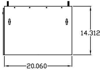
IQ14000V IQ17000V IQ20000V FRONT VIEW
