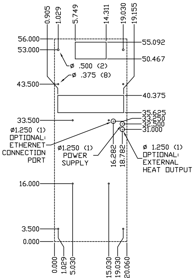
IQ14000V IQ17000V IQ20000V CUTOUT DRAWING
