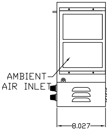
IQ1000V LEFT SIDE
