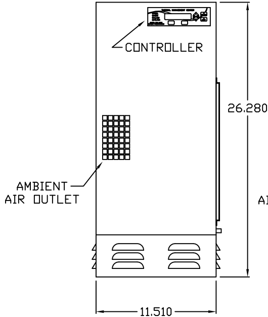
IQ1200VS IQ1500VS IQ1800VS FRONT VIEW
