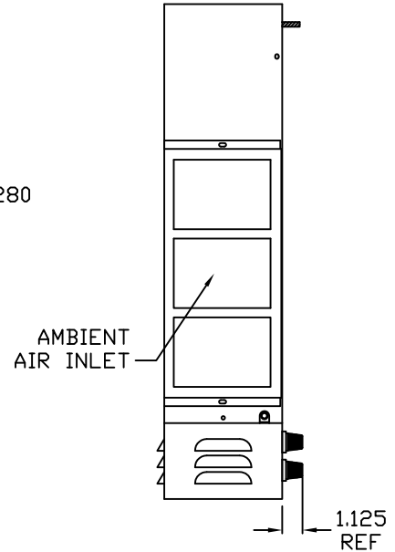
IQ1200VS IQ1500VS IQ1800VS RIGHT SIDE
