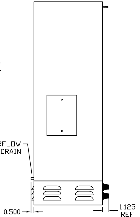
IQ1200VXS IQ1500VXS IQ1800VXS RIGHT SIDE
